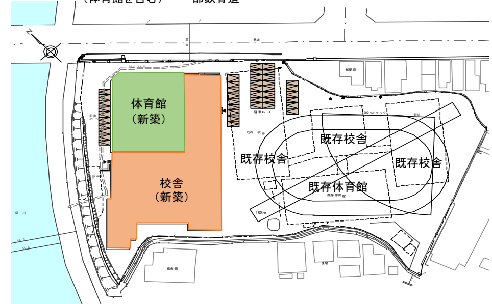
配置図
