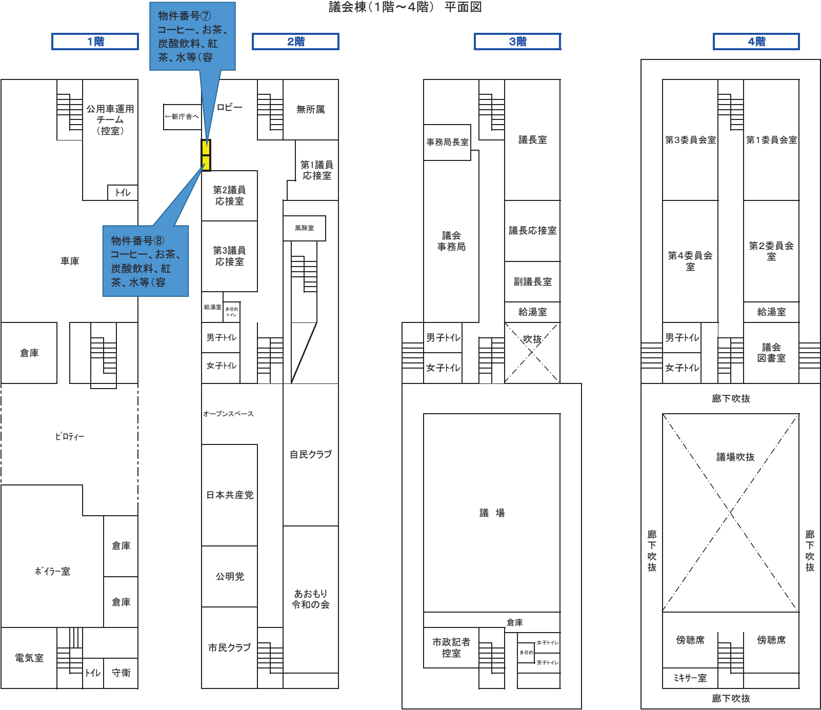
議会棟(1階～4階) 平面図
