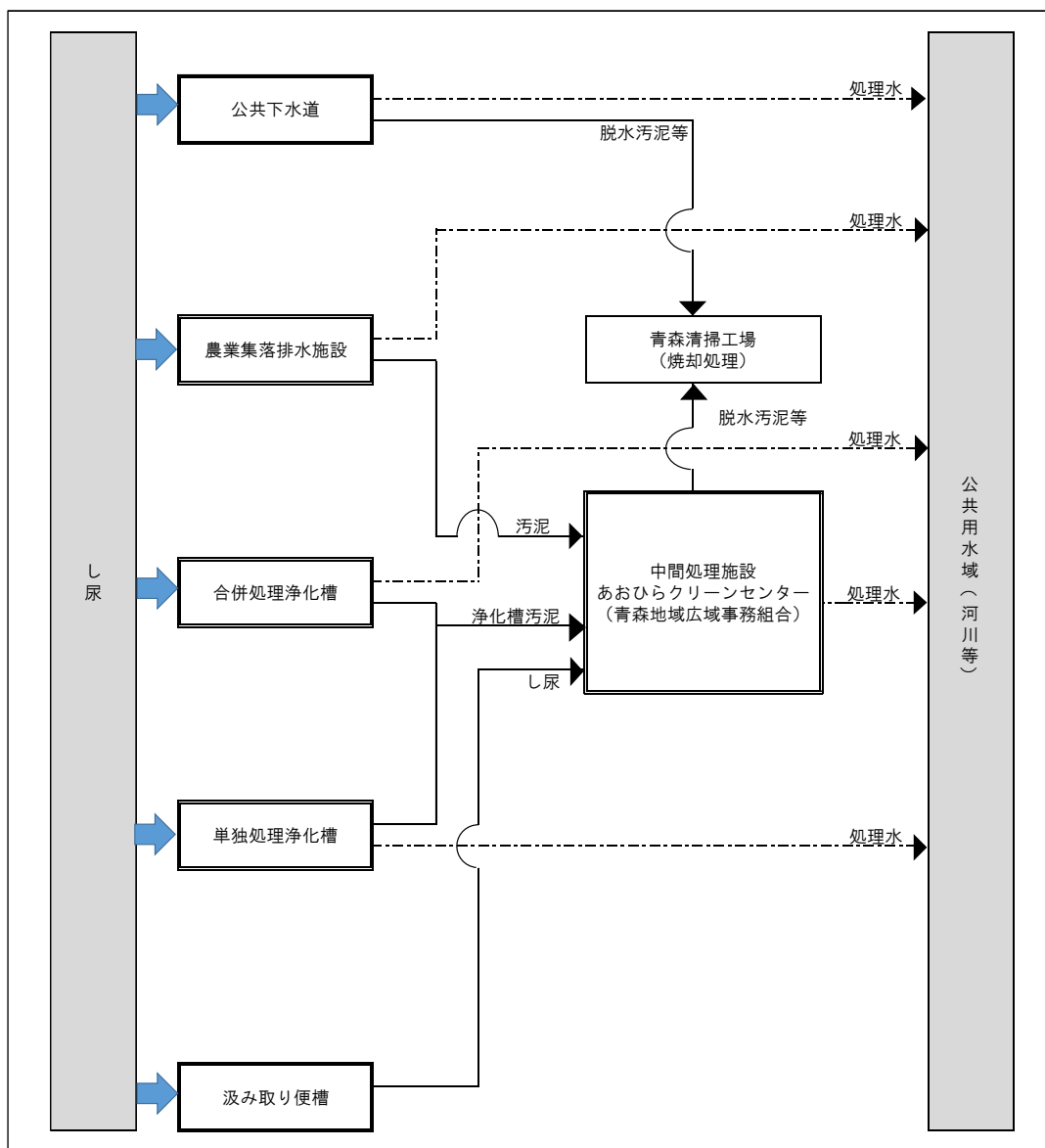
図3-1-1 生活排水処理の体系
