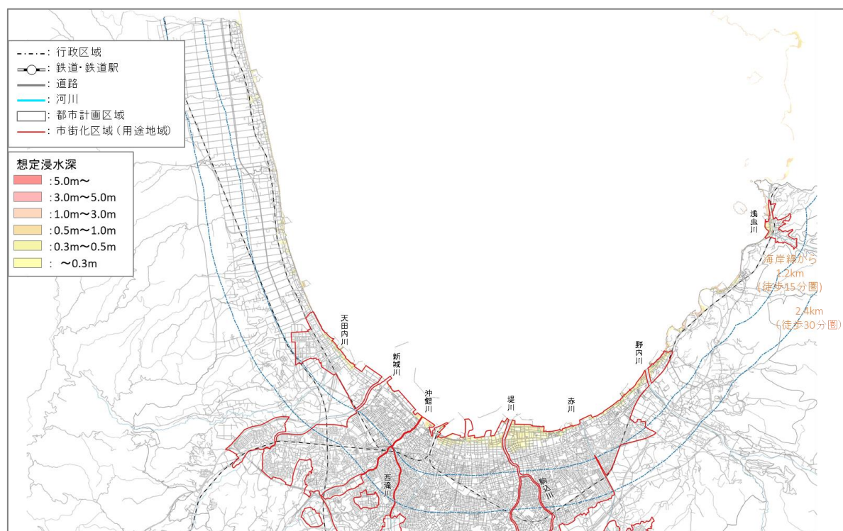
図 75 津波浸水想定区域（入内断層モデル）
