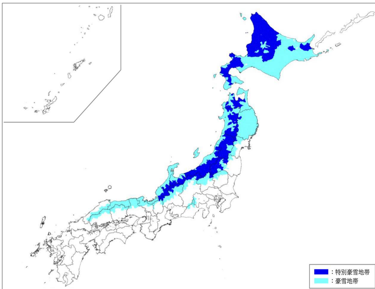
図 5 特別豪雪地帯及び豪雪地帯指定図
