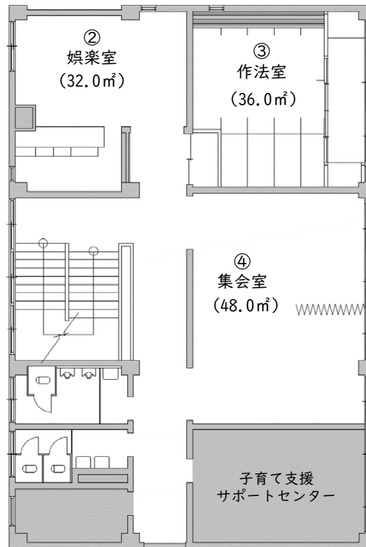
2階 平面図
