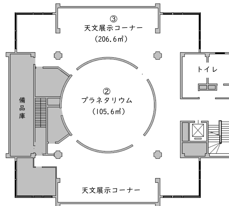
5階 平面図
