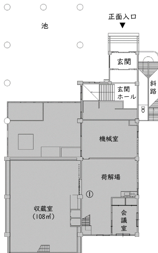
1階 平面図
