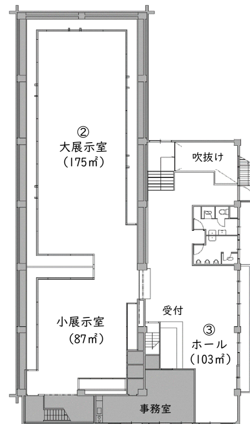
2階 平面図
