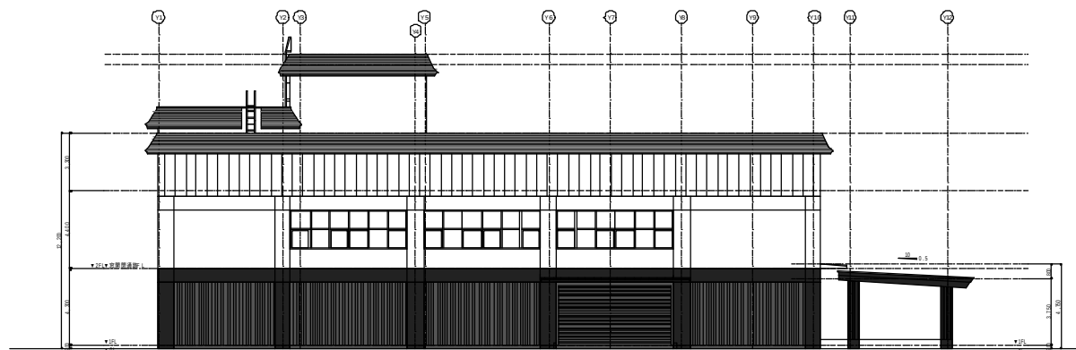
北側立面図 S=1/300
