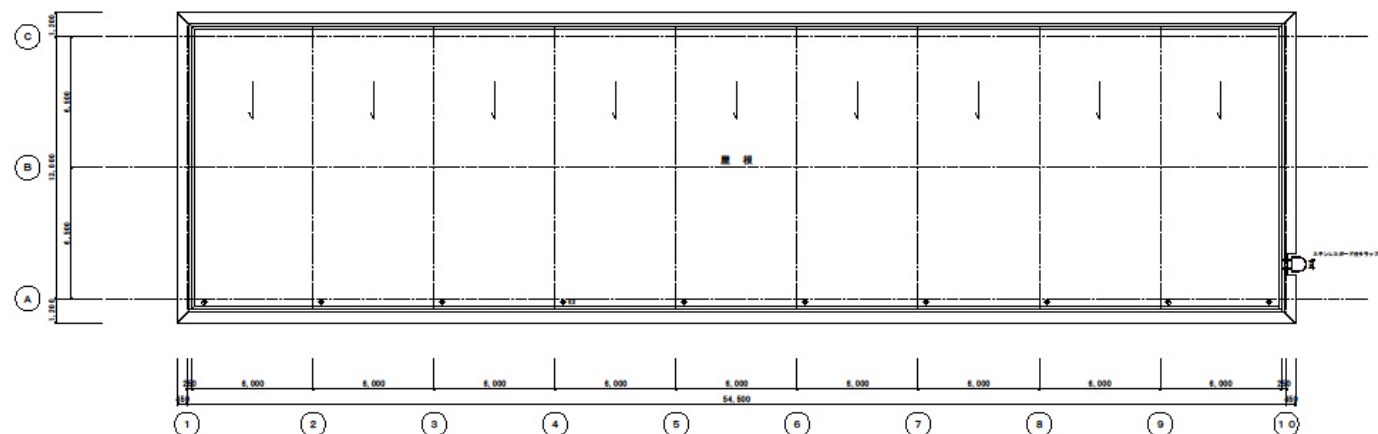
立面図 S=1/100
