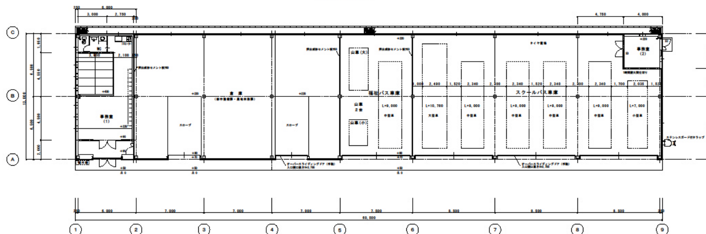
平面図 S=1/100
