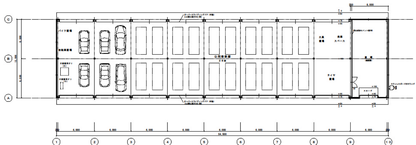
平面図 S=1/100
