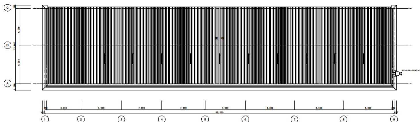
立面図 S=1/100
