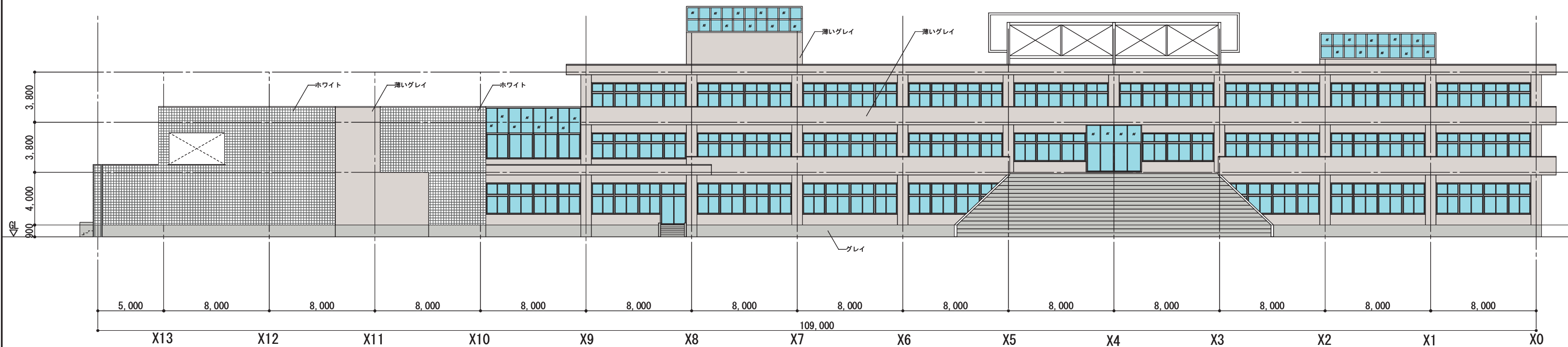
北側立面図 S=1:300
