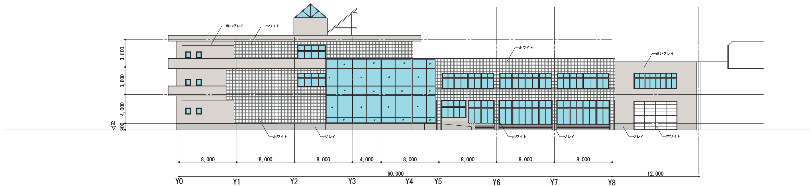
東側立面図 S=1:300
