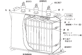
高圧コンデンサーの例
