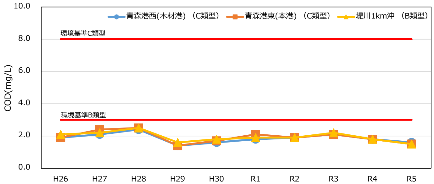
陸奥湾COD（75%値）経年変化
