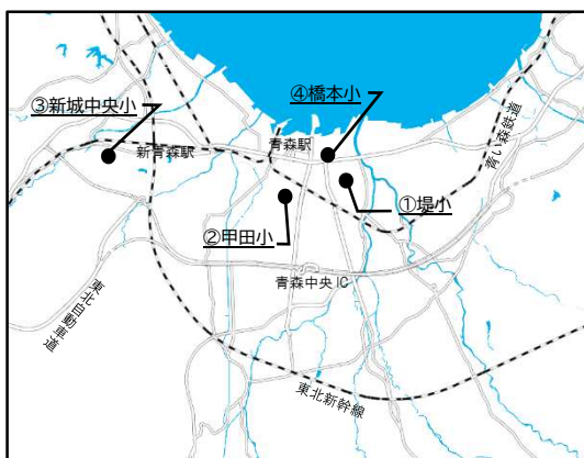
図 3-34 大気汚染測定地点（青森）
