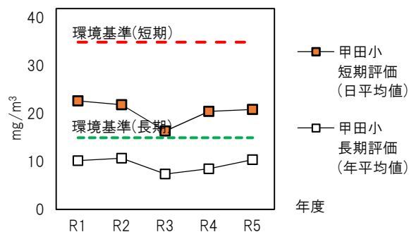
図3-41 微小粒子状物質の短期的評価及び長期的評価の推移
