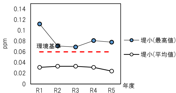
図3-38 光化学オキシダントの昼間の1時間値の推移
