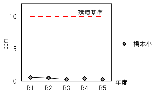
図3-39 一酸化炭素の年平均値の推移
