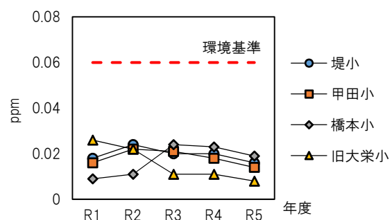
図3-37 二酸化窒素の日平均値の推移
