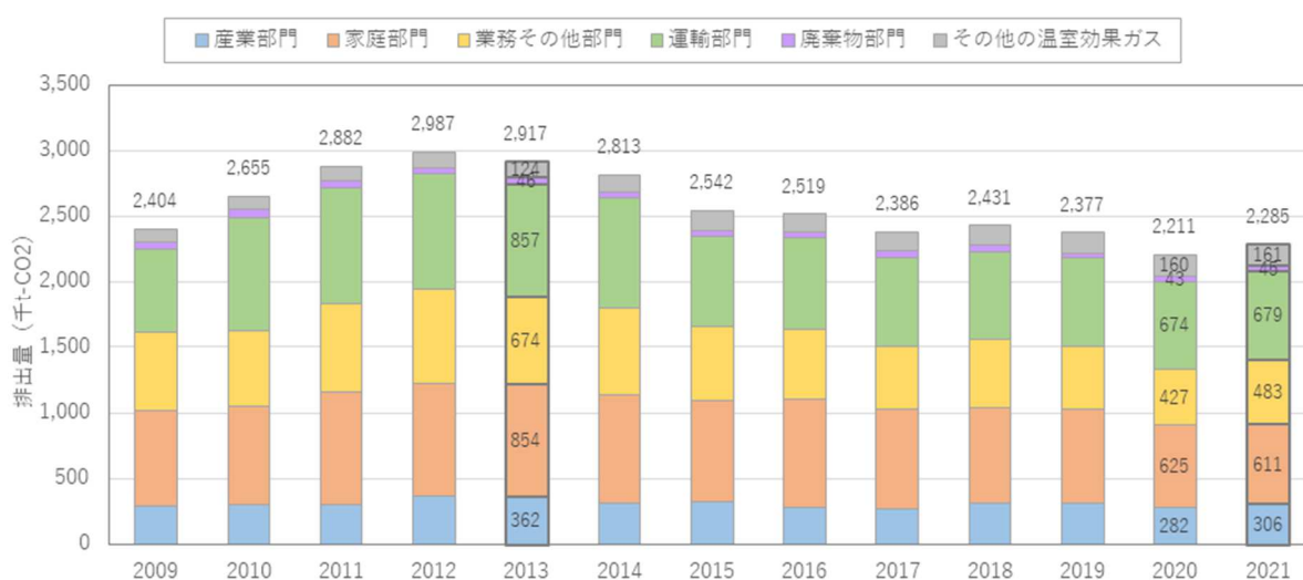
図 3-3 温室効果ガスの総排出量の推移
