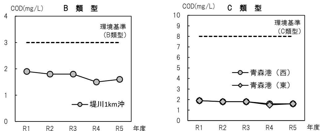
図 3-44 海域別（環境基準点）における COD（75%値）の経年変化
