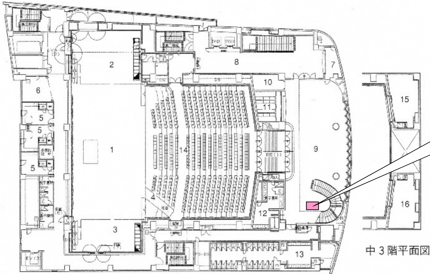
2階平面図 (演劇型式)
